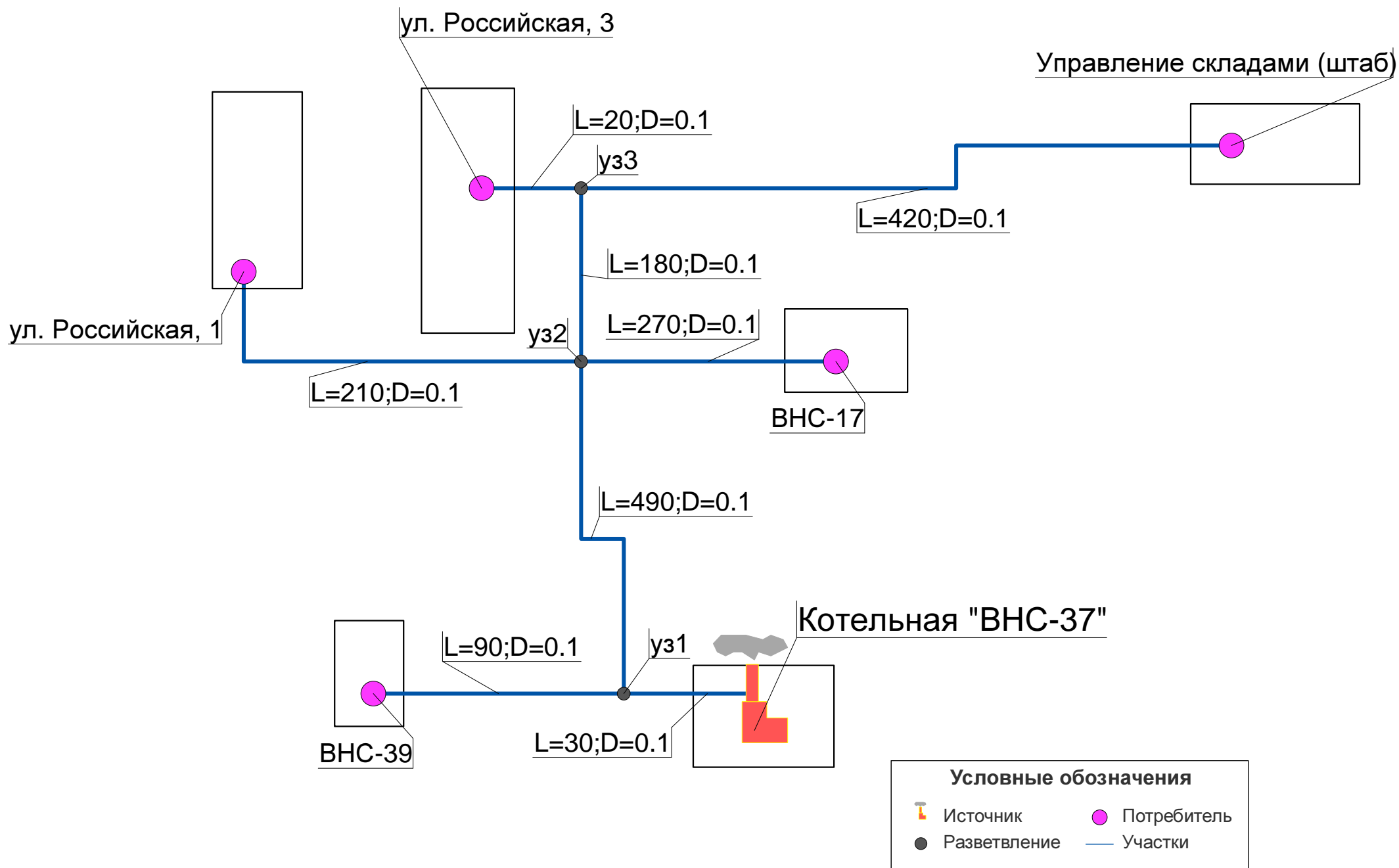
Рис.1. Схема тепловых сетей котельной "ВНС-37" МП "Новокручининское"
